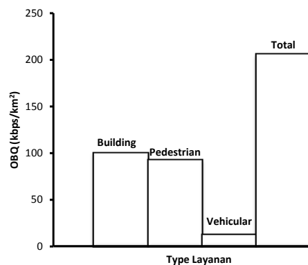
Gambar 4. OBQ Total Wilayah Suburban
