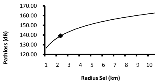
Gambar 5. Path Loss Wilayah Suburban Sebagai Fungsi Radius Sel
