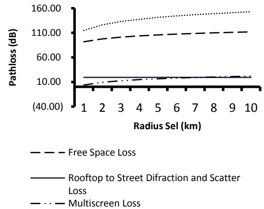
Gambar 6. Path Loss Wilayah Urban Sebagai Fungsi Radius Sel
